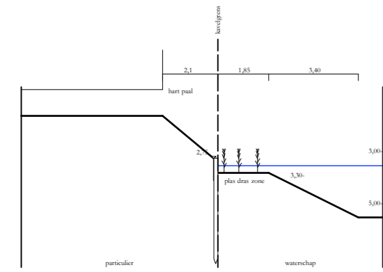
DOORSNEDE AA
